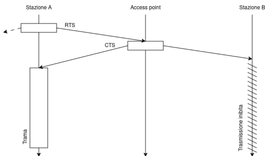
Figura 5.12: Funzionalità RTS-CTS
