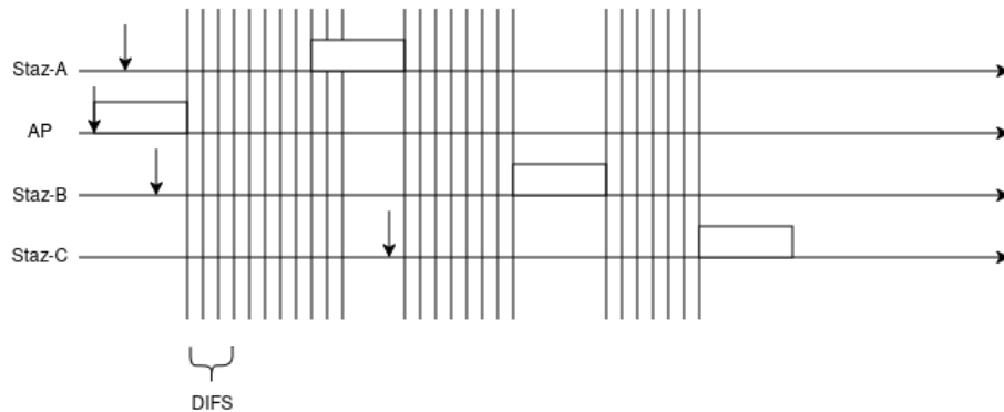
Figura 5.10: Algoritmo CSMA-CA
